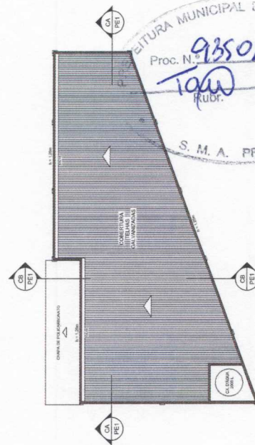
3 Cobertura 1:125
